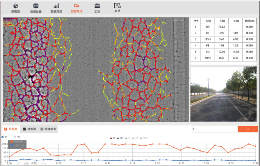
图-13 数据集成(裂缝宽度1~10mm标注图)
