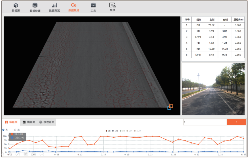
图-14 数据集成(10m损坏标注图)
