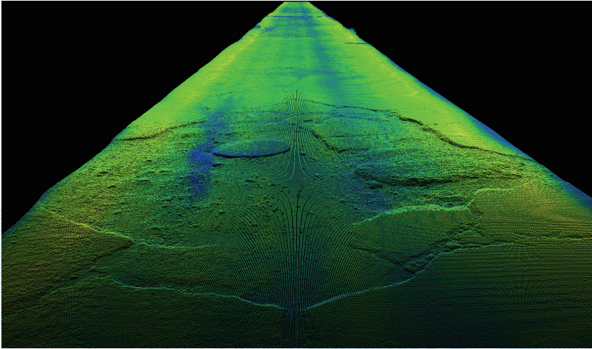
图-8 松散类损坏
